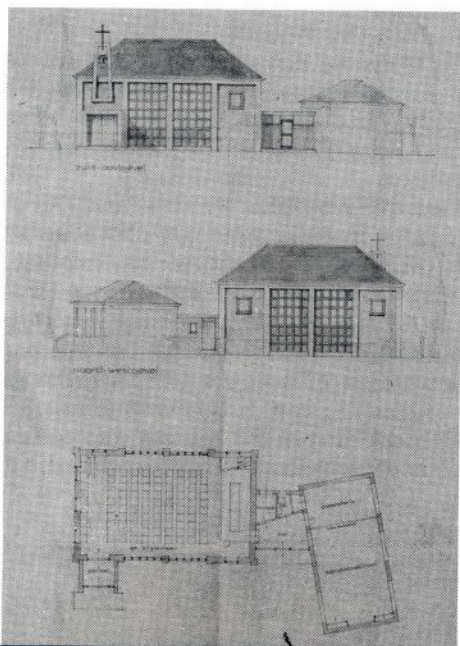
Schetsplan voor een te bouwen „verenigingslokaal” te gebruiken als kerk, door J.C. Swen te Bussum, 1952.
